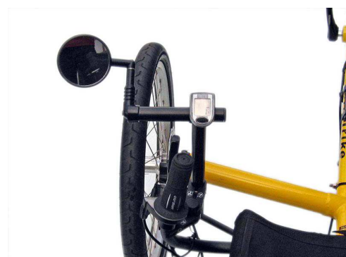
Cockpit Mount, Spiegel und Computerhalter montiert
